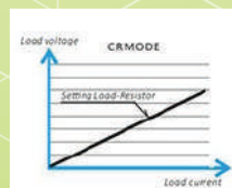
CR MODE
